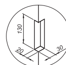
a falnyílás kialakítása 3 pántos ajtó tokhoz
