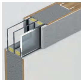
Háromrétegű meleg peremes üvegezéssel – P4 betörésvédelmi osztály, rozsdamentes acél kerettel
