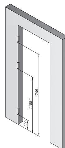
a falnyílás kialakítása 3 pántos ajtó tokhoz
